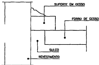
Detalhe - Junta de Dilatação Sem Escala
