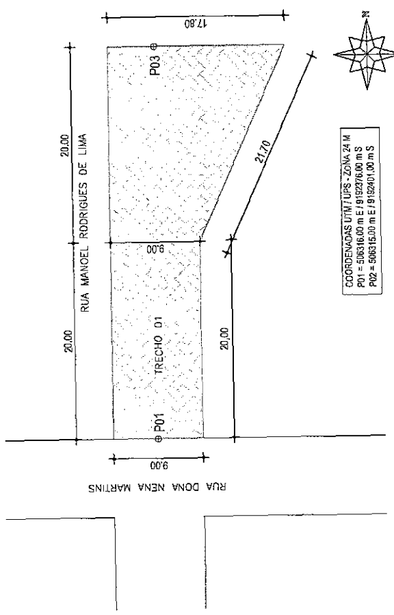
PLANTA BAIXA DE PAVIMENTAÇÃO ESC: 1/125
