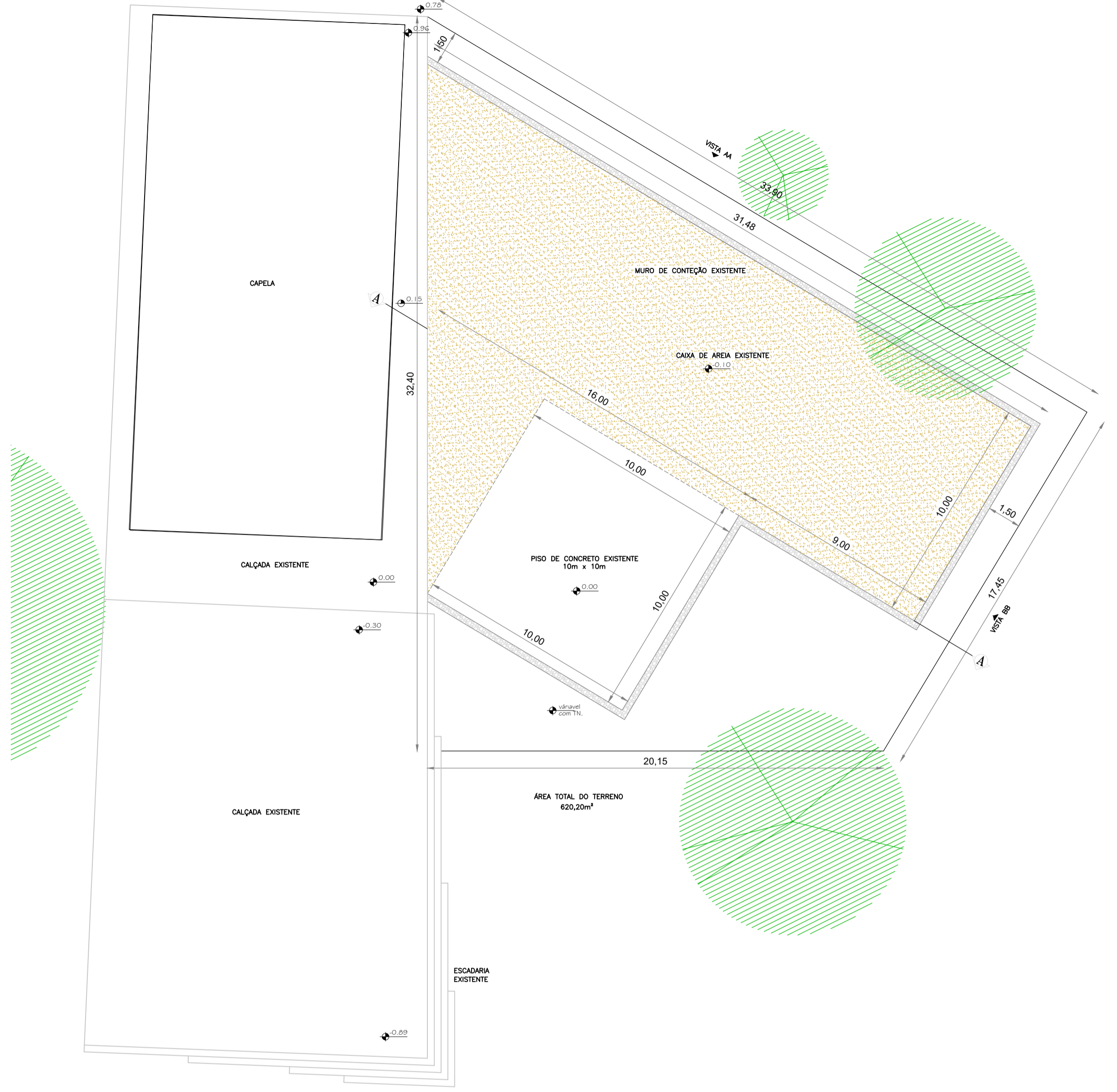
PLANTA BAIXA EXISTENTE ESC.: ..... 1/150
