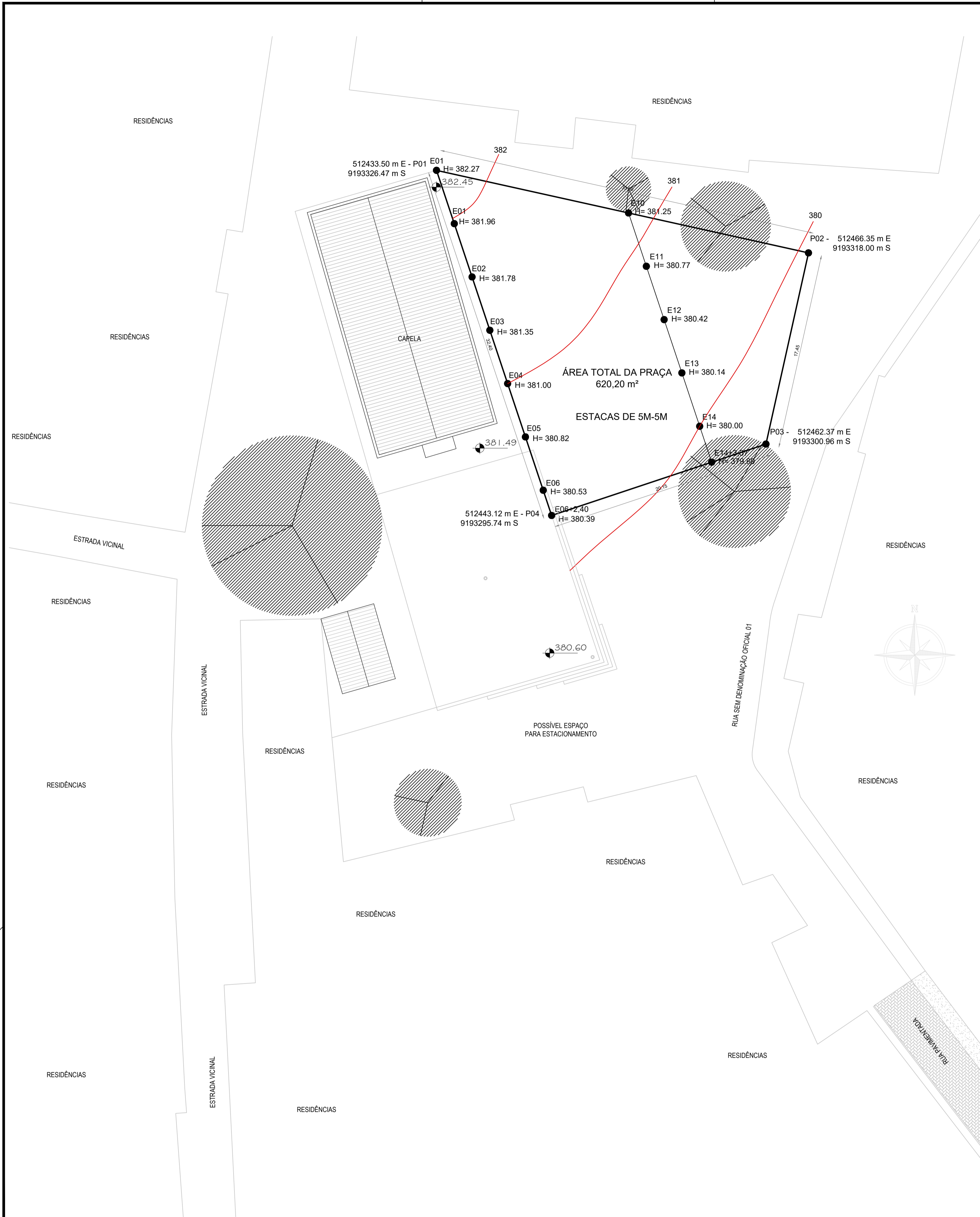
LEVANTAMENTO PLANIALTIMÉTRICO ESC.: ..... 1/200
